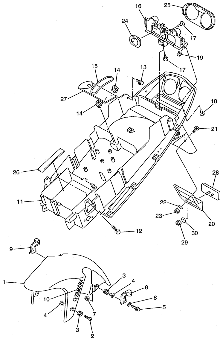
FIG. 21 GUARDABARRO
