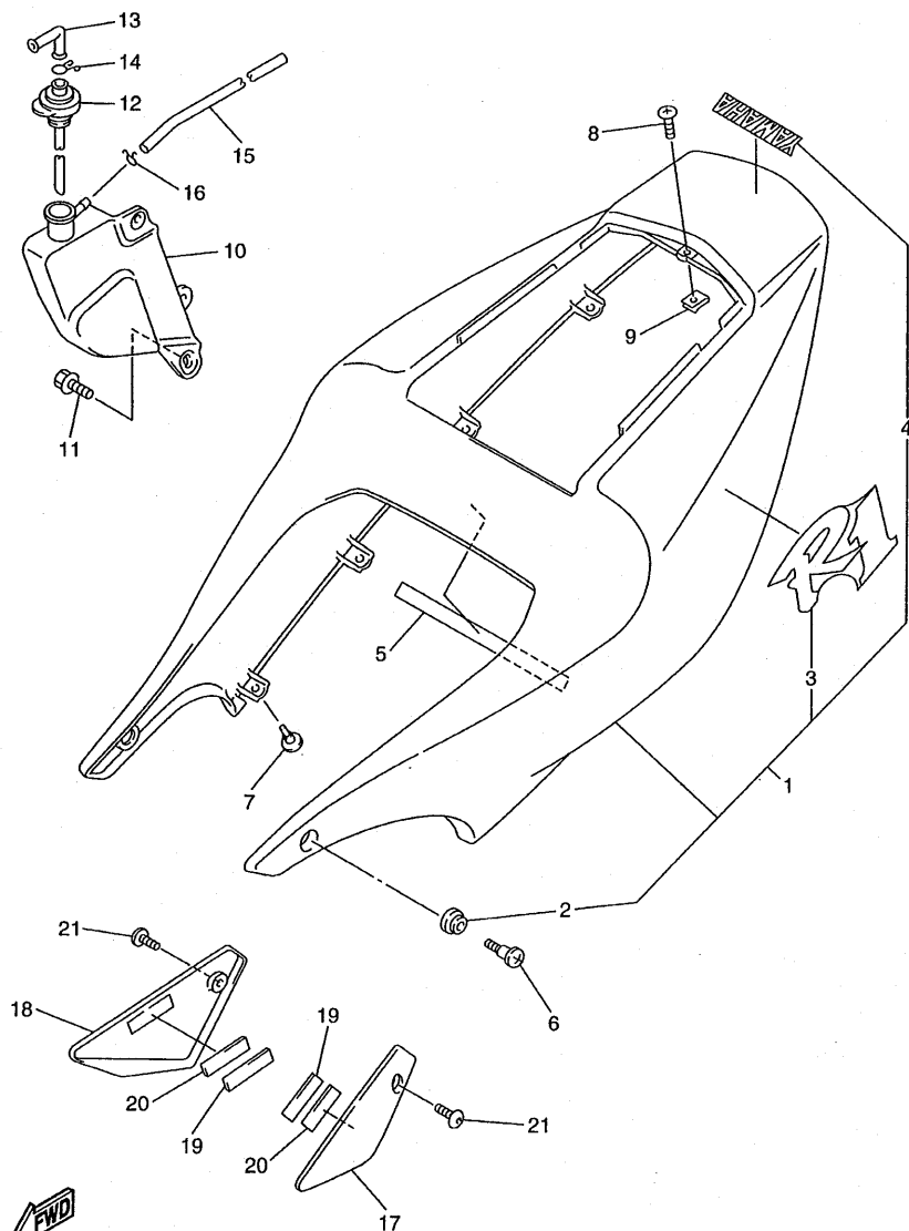
FIG. 22 CUBIERTA LATERAL
